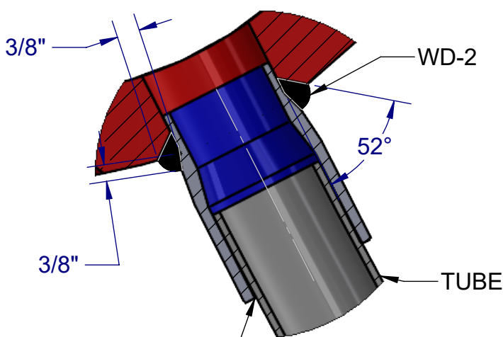
WD-1 DETAIL B SCALE 1 : 2
